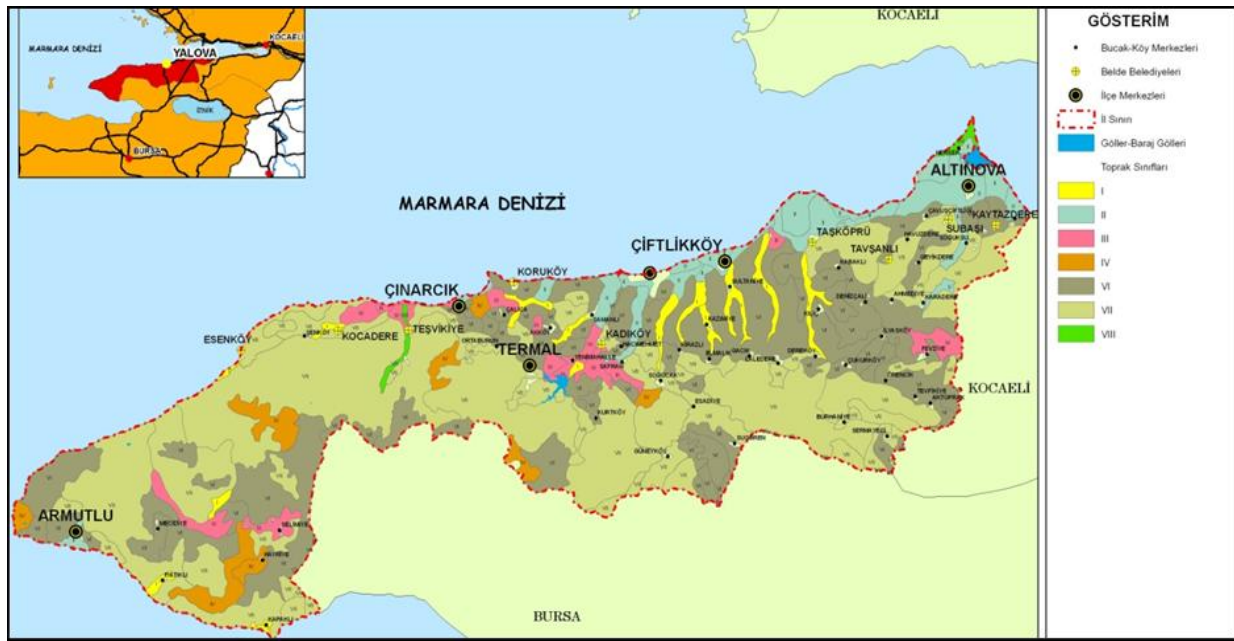
Şekil 7: Yalova İli Toprak Sınıfları
