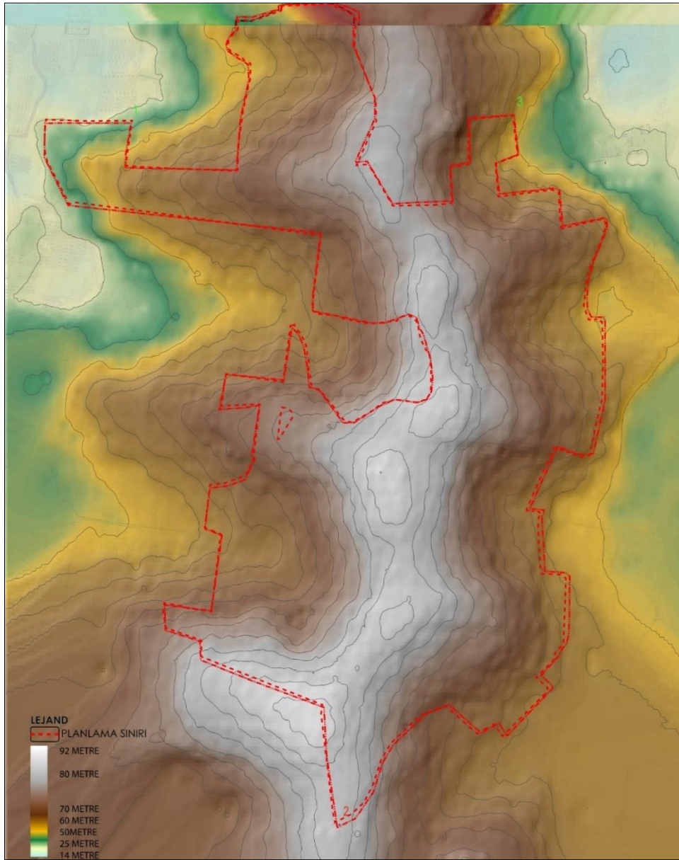
Harita 5: Eşyüksekti Analizi Haritası
